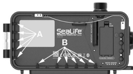
Vooraf geïnstalleerde rubberen greeplipjes van gemiddelde grootte (A)
